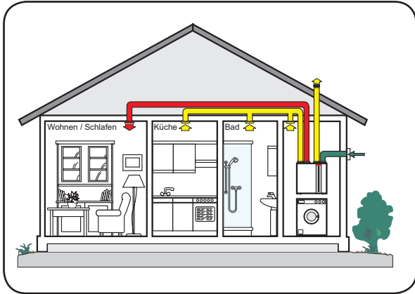
Bild 2: Zentrales System mit Wärmeübertrager
