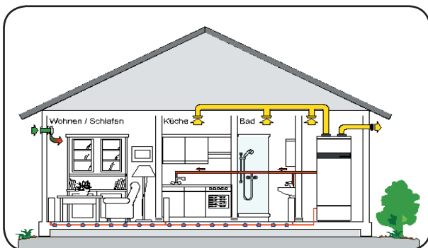
Bild 3: Zentralsystem für Abluft mit Wärmerückgewinnung und Wärmeaustauscher
