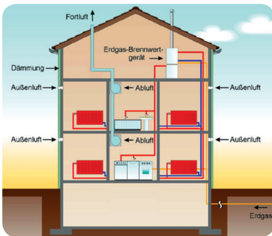
Bild 5: Dezentrale Abluftanlagen mit Zuluftelementen ohne Wärmerückgewinnung
