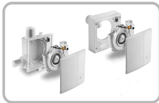
Bild 5: Dezentrale Abluftanlagen mit Zuluftelementen ohne Wärmerückgewinnung
